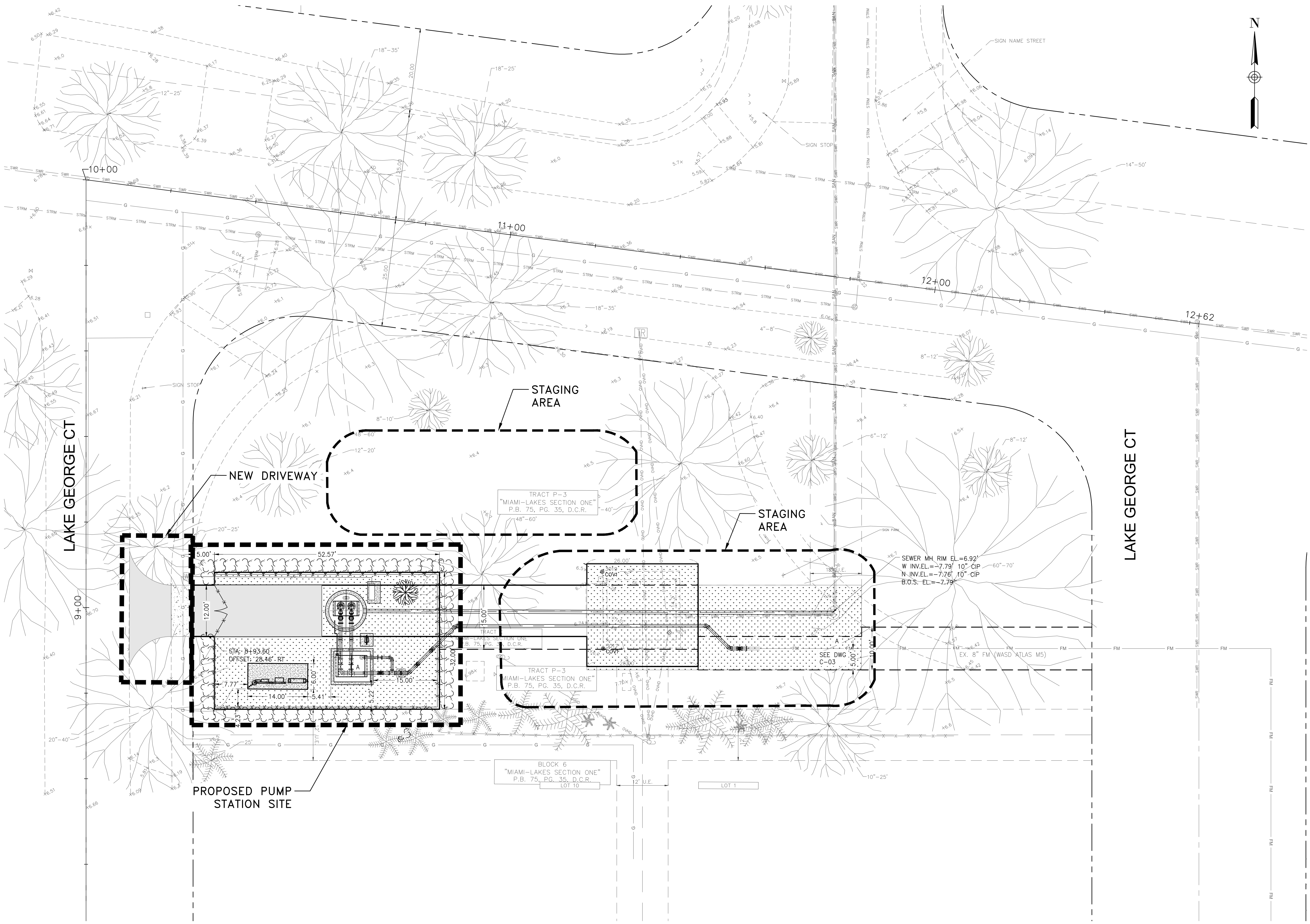
SITE LAYOUT SCALE: 1"=10'-0"
